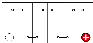
Schaltung 0
